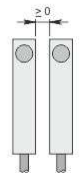
Montaje lateral
